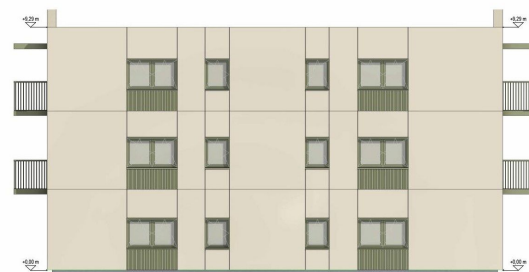
ELEWACJA 4
